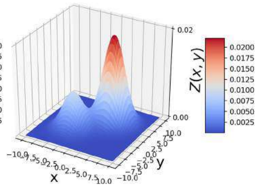
(d) \pi_1 = 0.3, \pi_2 = 0.7
