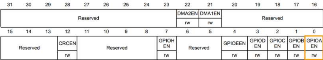
Figure 2.15: RCC AHB1 ER
